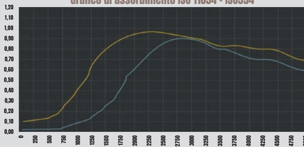
9 mm 1200 gr/m 2 - Feltro acustico - Rivestimento MDF Grafico di assorbimento ISO 11654 - ISO354
